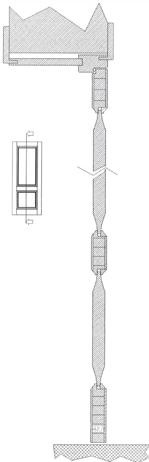
Coupe verticale d'une porte intérieure avec paumelles invisibles AGB Eclipse
