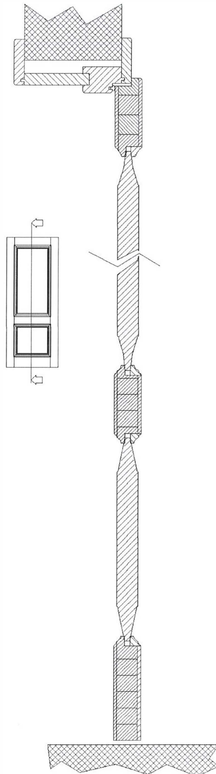
Coupe verticale d'une porte intérieure avec paumelles cylindriques
